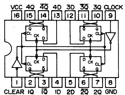
74LS273
