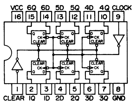
74LS174
