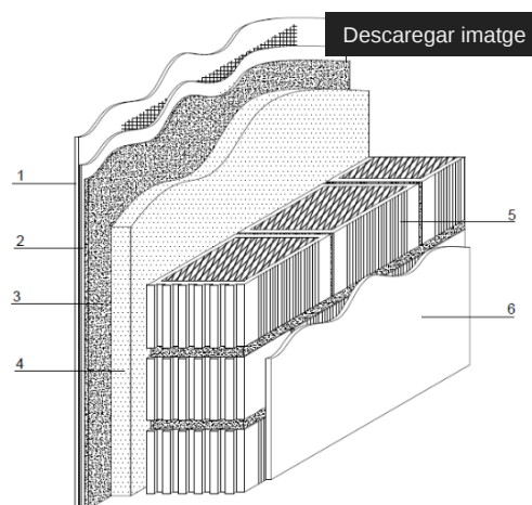
Detalle 2. Sección Fachada Tipo 2 [Fuente propia]
